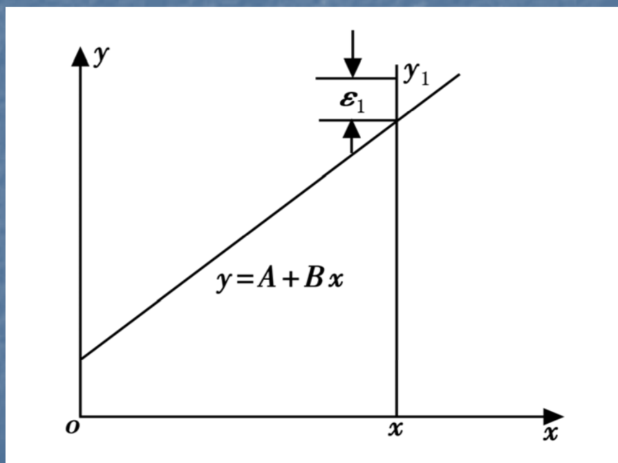
图1-2 直线 y=A+Bx
