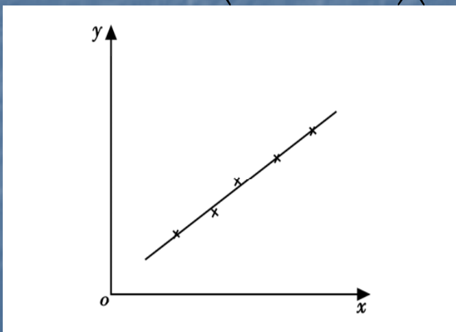
图1-3 密集分布(r值接近于1)
