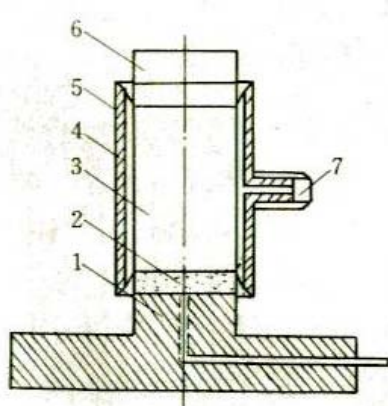
图 16.2.1-5 原状土切土盘分样器
