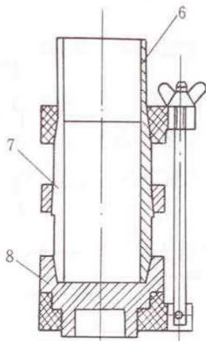
图 16.2.1-2 击样器
