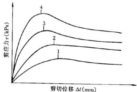
图 18.1.5 剪应力与剪切位移关系曲线
