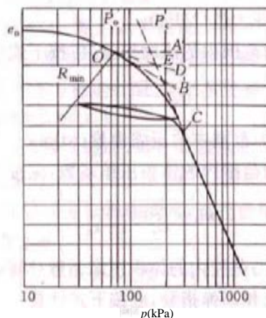
图 14.1.14 e-\log p 曲线求 p_c 示意
