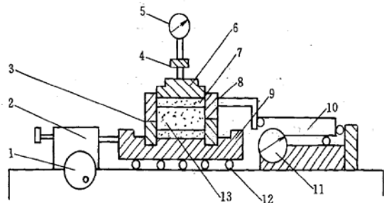
图 18.1.2 应变控制式直剪仪
