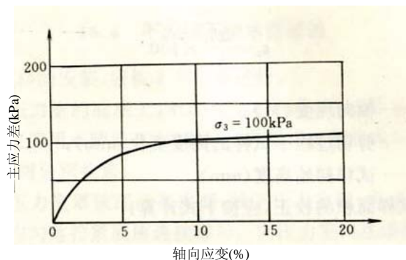
图 16.4.6 主应力差与轴向应变关系
