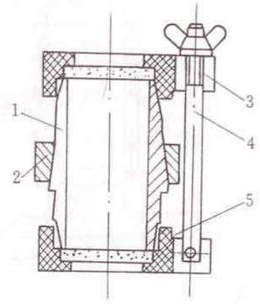
图 16.2.1-3 饱和器
