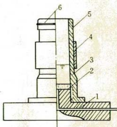
图 16.2.1-6 原状土切土盘分样器
