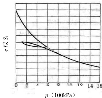
图 14.1.13 e(S_v)-p 关系曲线
