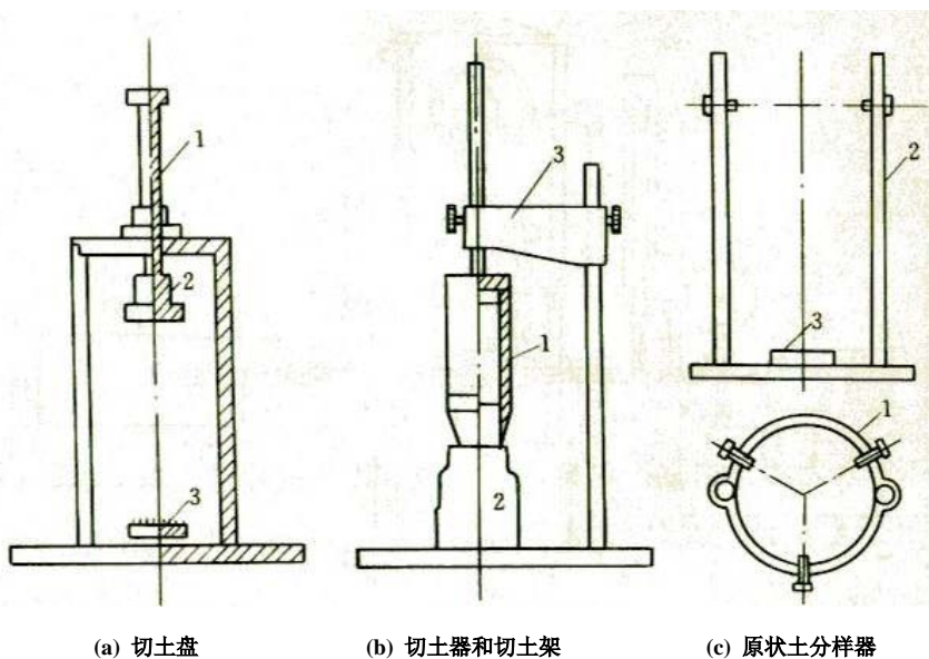
图 16.2.1-4 原状土切土盘分样器
