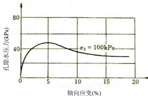
图 16.5.12 孔隙水压力与轴向应变关系曲线
