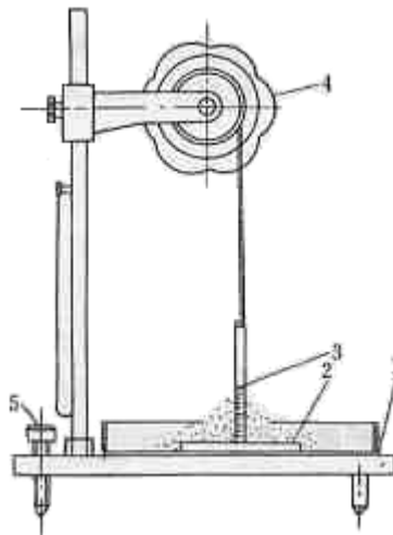
图 2.0.1 休止角测试仪
