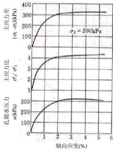
图 16.7.3 固结不排水剪应力应变关系
