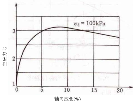
图 16.5.11 有效应力比与轴向应变关系曲线
