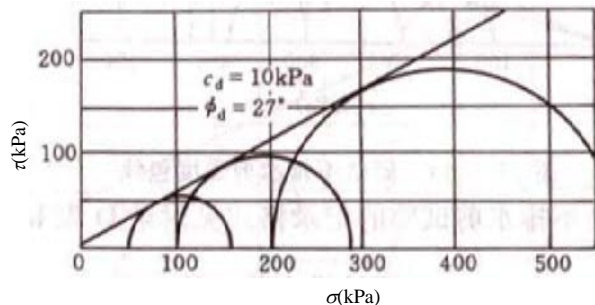
图 16.6.9 固结排水剪强度包线
