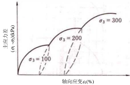
图 16.7.2 不固结不排水剪的应力-应变
