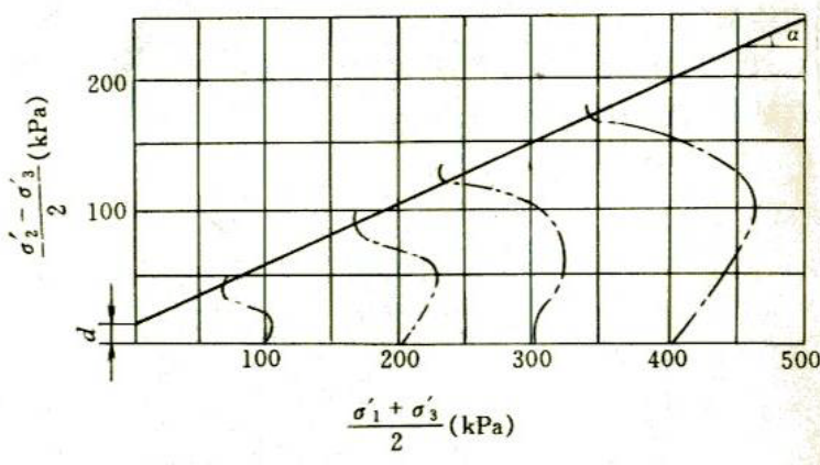
图 16.5.13 应力路径曲线
