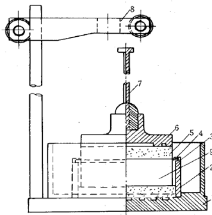
图 14.1.2 固结仪示意图
