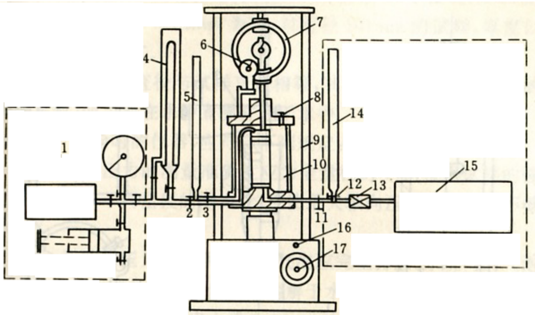
图 16.2.1-1 应变控制式三轴仪
