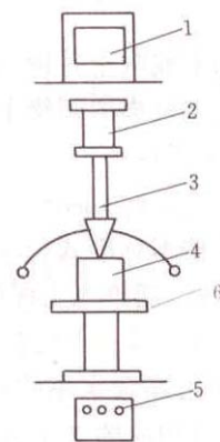
图 8.1.2 液、塑限联合测定仪示意图 1—显示屏；2—电磁铁；3—带标尺的圆锥仪； 4—试样杯；5—控制开关；6—升降座
