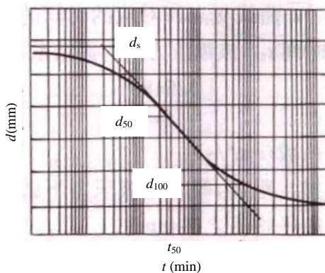
图 14.1.16-2 时间对数法求 t_{50}
