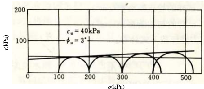
图 16.4.7 不固结不排水剪强度包线
