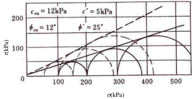
图 16.5.14 固结不排水剪强度包线
