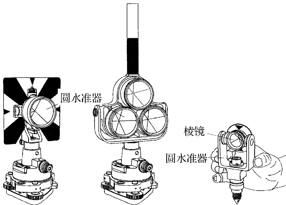
(a)单棱镜与基座 (b)三棱镜与基座 (c)ADSmin102 微型棱镜
