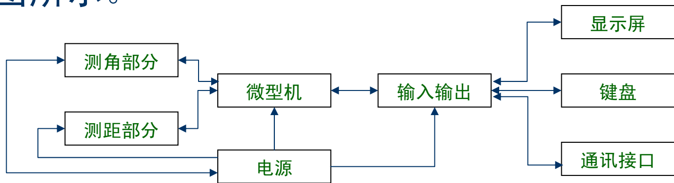
全站仪结构框图
