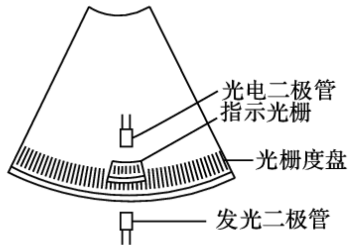
光栅度盘
