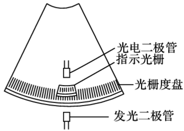
光栅度盘
