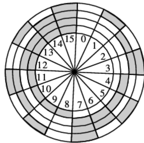
编码度盘
