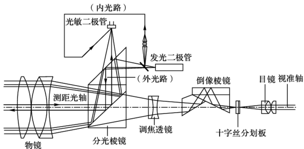
全站仪轴系及光路
