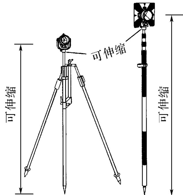
(a) 对中杆
